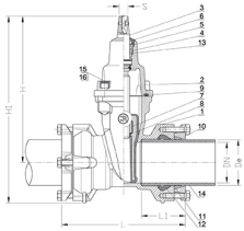
DuraGrip-muhviventtiilin mittakuva
